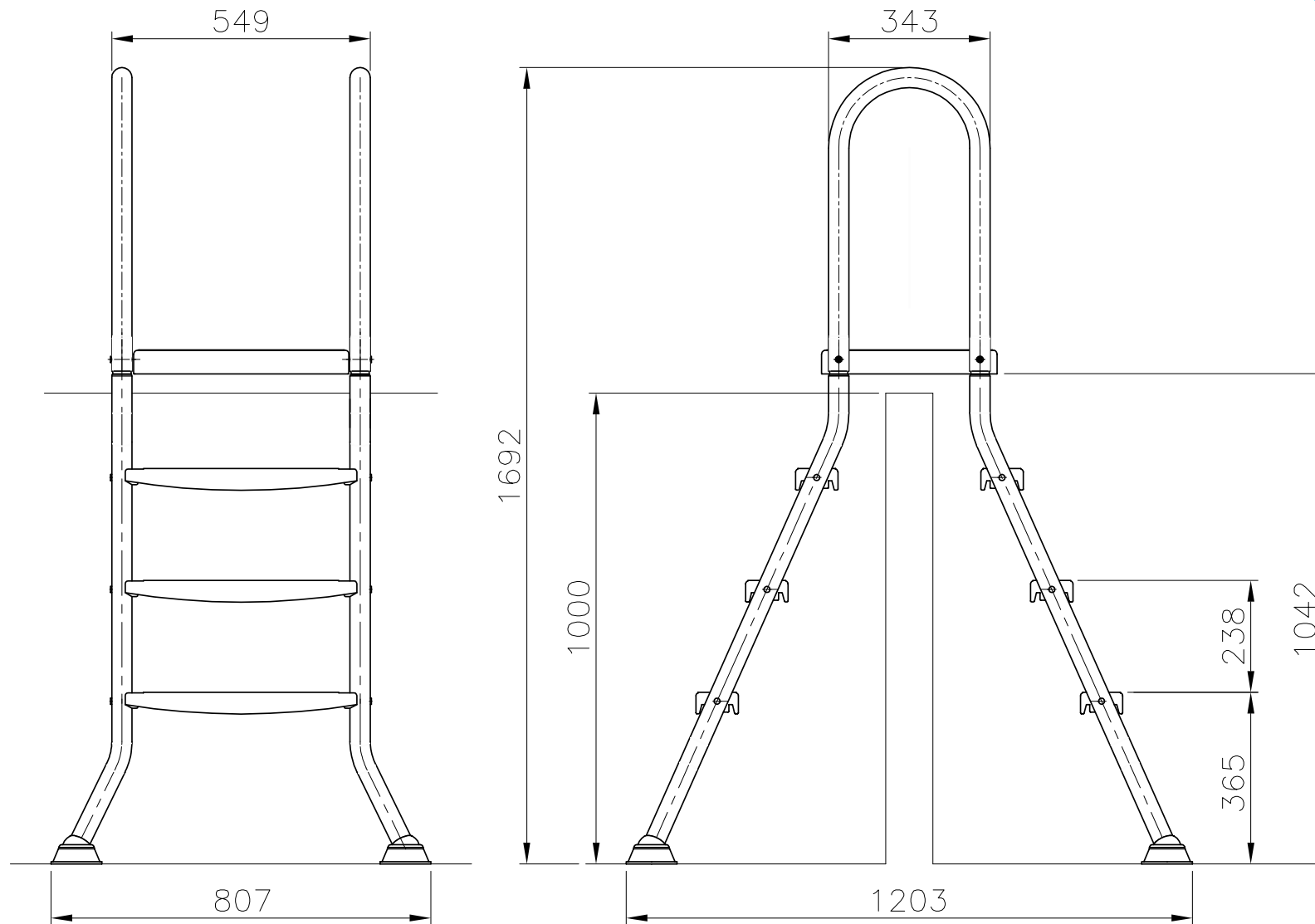
Edelstahl Aufstellbecken-Leiter für Becken bis 0,90 m Höhe
